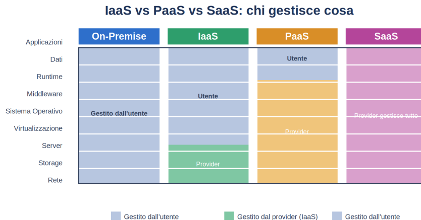
Figura 2 – Ripartizione delle responsabilità tra utente e provider nei tre modelli
